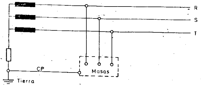
Fig. 8 Esquema IT con Toma de Tierra Común
