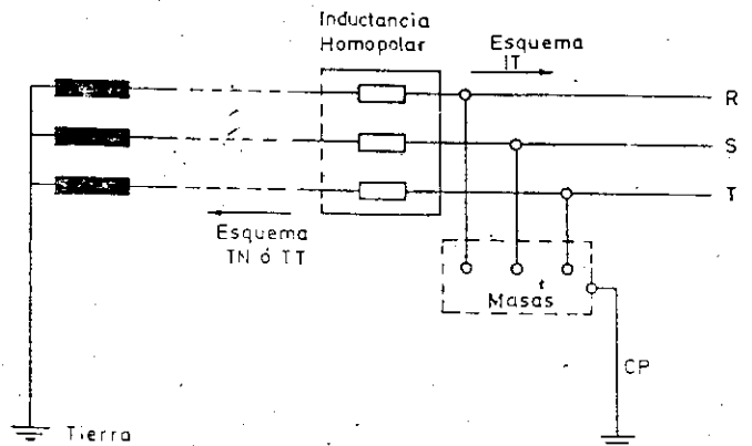
Fig. 9 Esquema IT en Serie con un Esquema TN o TT
