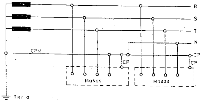
Fig. 4 Esquema TN-C-S
