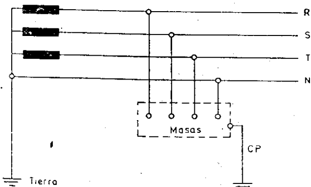
Fig. 6 Esquema TT
