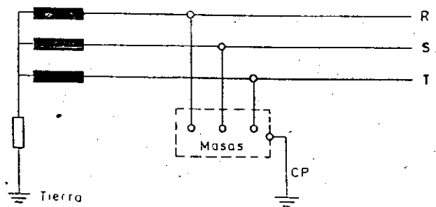
Fig. 7 Esquema IT con Tomas de Tierra Independientes
